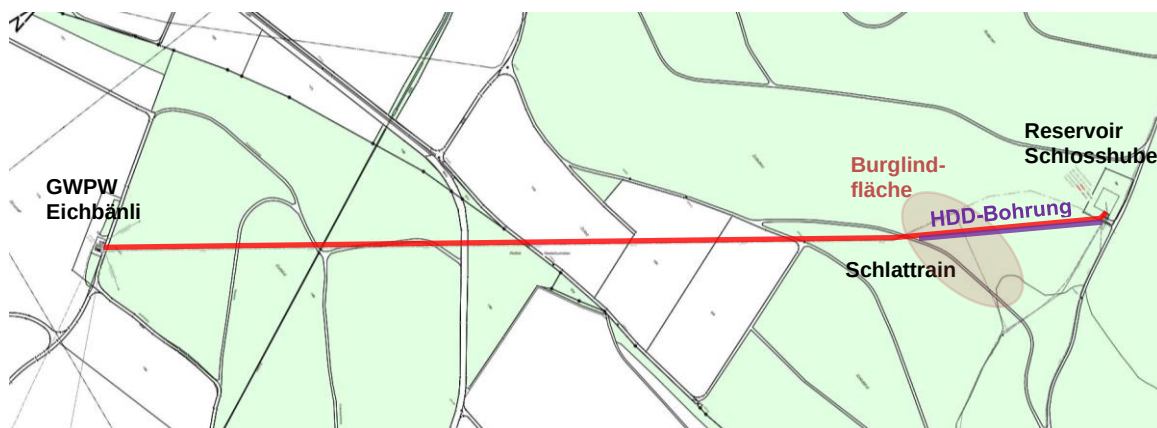
Abbildung 7: Linienführung Abschnitt 1 "Reservoir Schlosshubel – GWPW Eichbänli", Variante B
