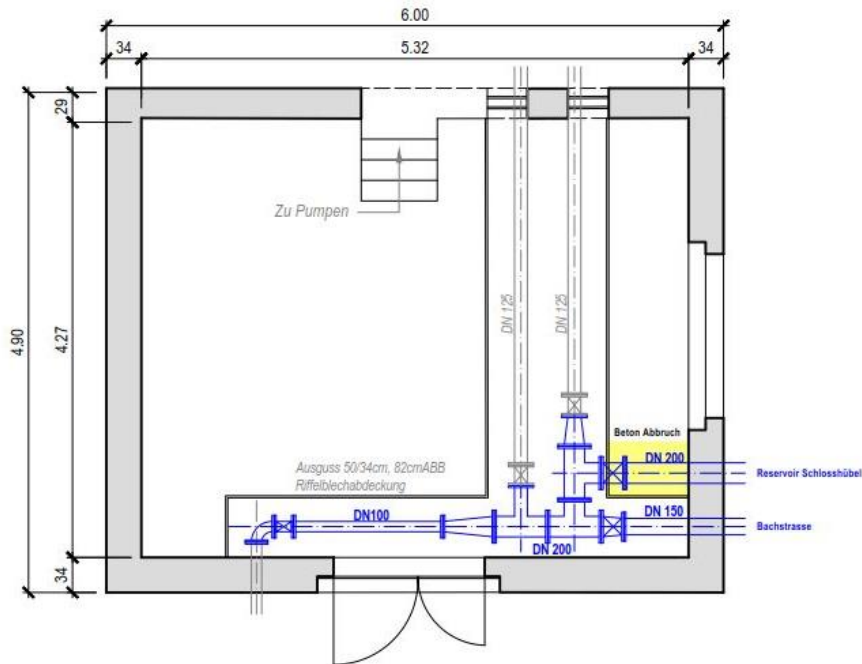
Abbildung 13: Anpassungen, Rohrkeller GWPW Eichbänli, neue Grossrohrinstallation (blau)
