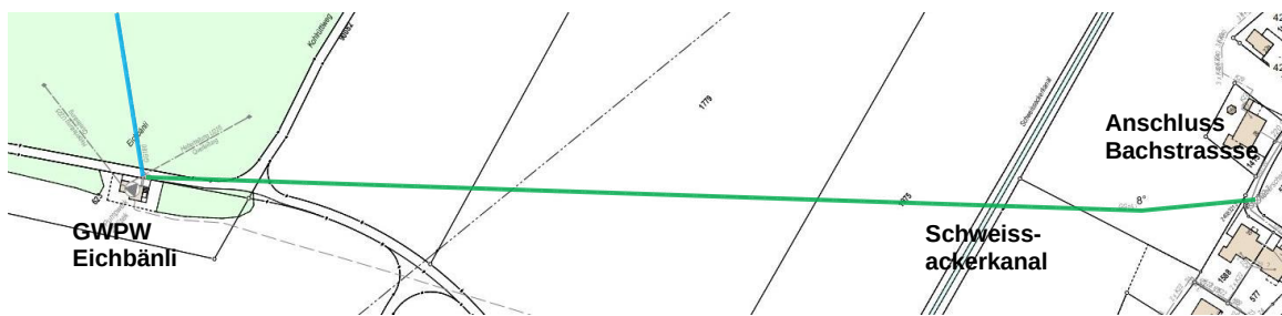
Abbildung 5: — Leitung "GWPW – Bachstrasse" — Leitung "Reservoir – GWPW"
