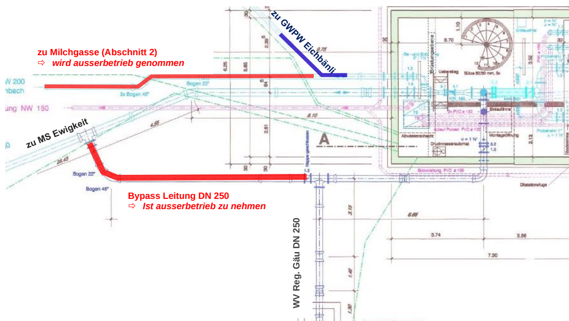
Abbildung 12: Ausschnitt PdaB Reservoir schlosshubel, 28.10.2013, Grundriss Rohrkeller
