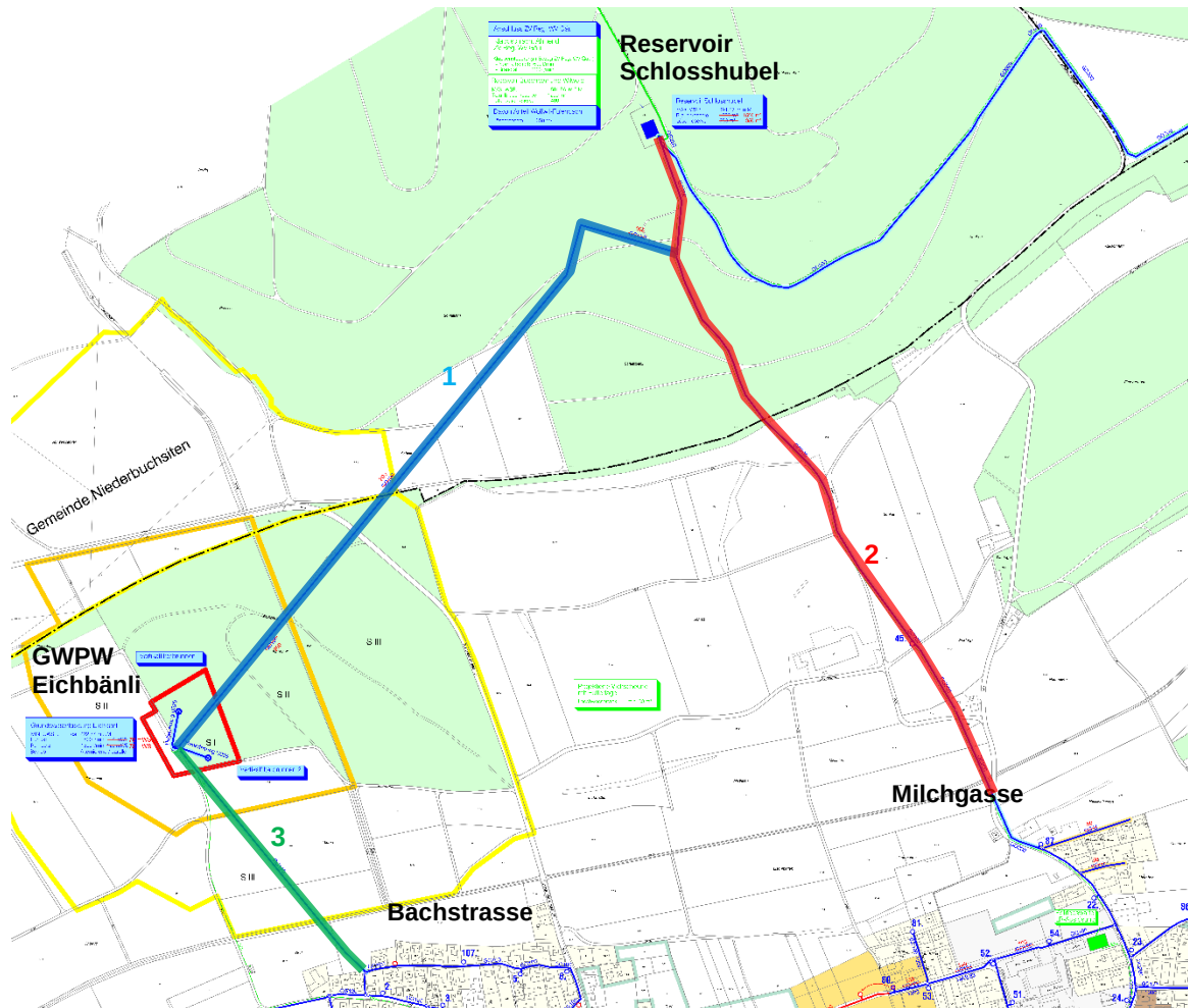
Abbildung 2: Ausschnitt aus GWP Wolfwil (RRB 182, 19.02.2013), Geplanter Leitungsersatz farblich markiert
