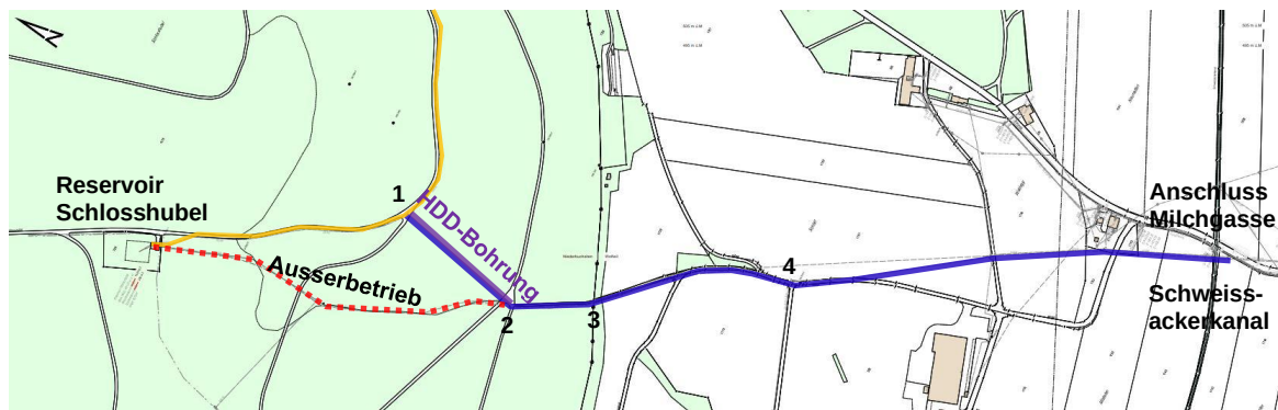
Abbildung 10: Neue Linienführung Abschnitt 2 "Reservoir Schlosshubel – Milchgasse"
