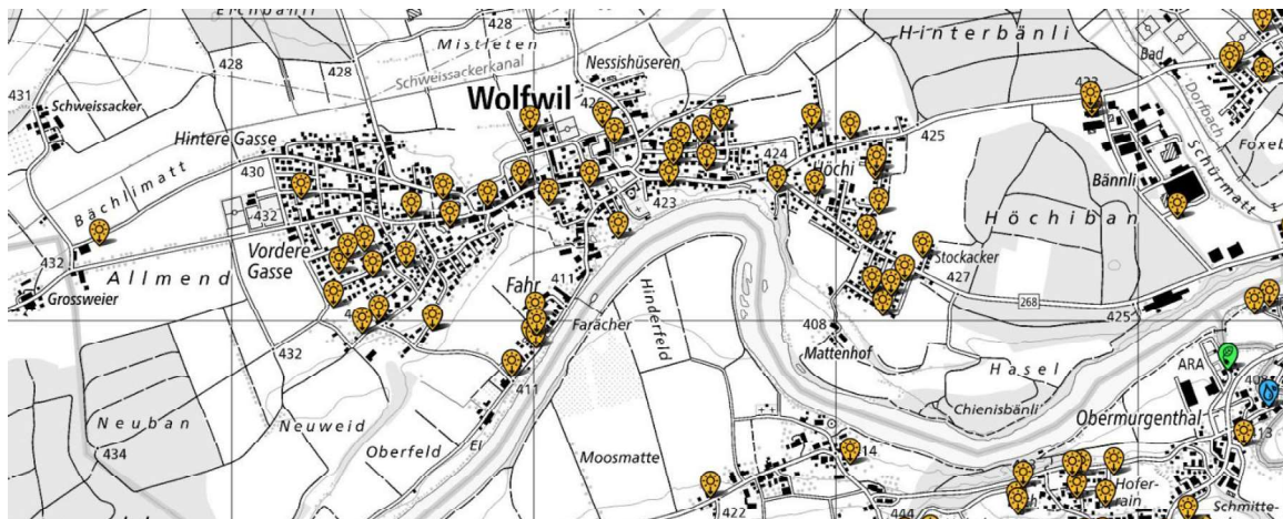
Übersicht Elektrizitätsproduktionsanlagen
